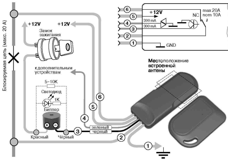
Схема подключения иммобилайзера Stealth 477
